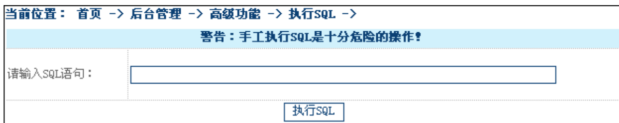
图 13.3 执行 SQL
